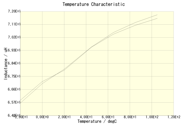
CLF10040T-680M-CA(DC = 0A)
